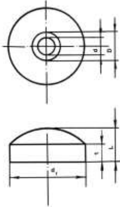
Рис. 1. Шаблон для определения достоинства пробойн
