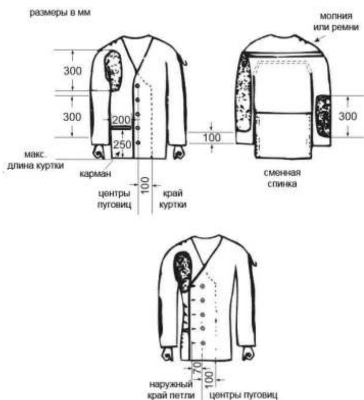
Рис. 1. Стрелковая куртка
