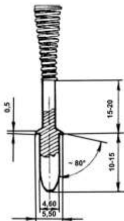
Рис. 1. Наружный калибр для определения достоинства пробойны в стрельбе из пневматической винтовки
